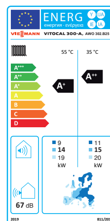
Energetický štítek Vitocal 300-A, AWO 302.B25
